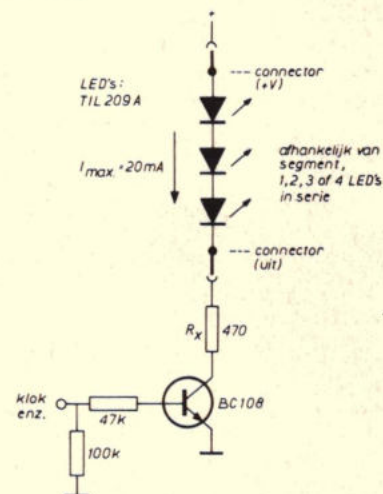
Fig. 4. LED-sturing. Omdat een MOS circuit geen 20 mA mag voeren, is deze buffer per segment vereist.
